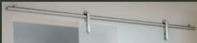
DORMA RSP 80 Glas zur Wandmontage Glasgewicht (kg): max. 80 kg 8 und 10 mm ESG Aluminiumfarben
